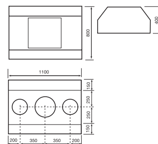
Размеры THM
