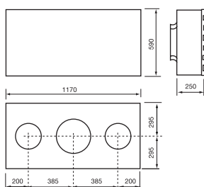
Размеры VGM
